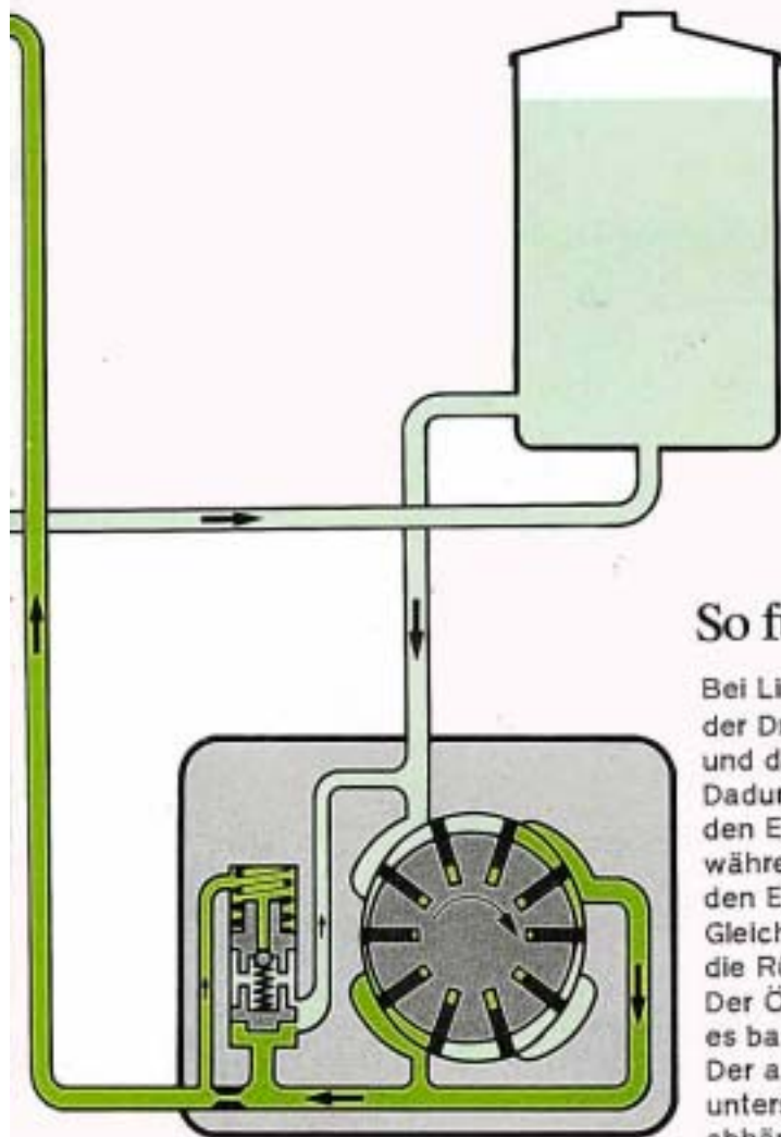
Flügelzellenpumpe
