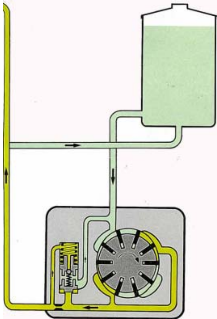
Flügelzellenpumpe
